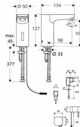
01 229 06 99 SCHELL Celis E, mezclador, alimentación a baterías 9 V.
