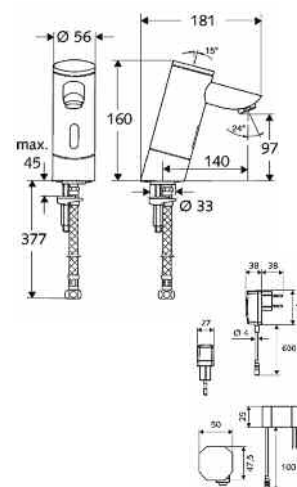
01 201 06 99 SCHELL Puris E, mezclador, alimentación a batería 9 V.
