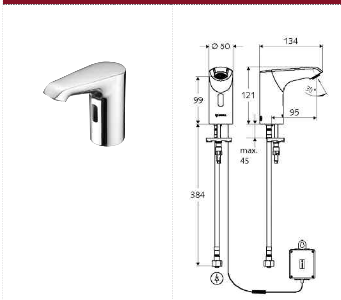
01 204 06 99, 00 224 06 99 SCHELL Xeris E Small, 1 agua, alimentación a red.
