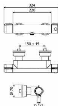
02 185 06 99 SCHELL MODUS Grifería de ducha termostática
