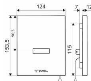
00 230 15 99, 00 230 06 99, 00 231 28 99 SCHELL Edition E, escudo electrónico sin contacto
