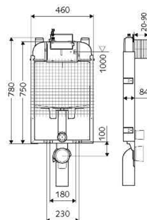
03 059 00 99 SCHELL cisterna con bastidor MONTUS C-N 80 para obra de fábrica DN 15 R 1/2".
