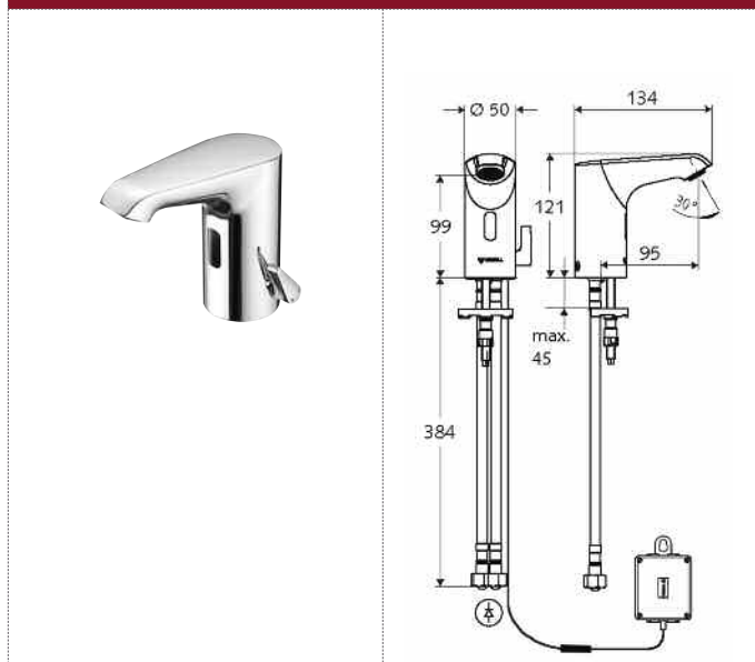
00 227 06 99, 01 210 06 99 SCHELL Xeris E Small, mezclador, alimentación a red.
