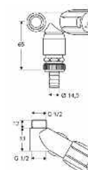
03 351 06 99 SCHELL grifo COMFORT para conexión de manguera.
