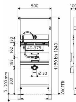
03 089 00 99 Bastidor Compact II LC, para montaje del sistema electrónico invisible Compact LC
