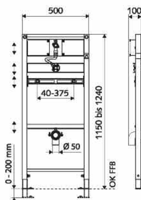
03 075 00 99 SCHELL bastidor Compact II con fluxor empotrado supersilencioso DN 15 G 1/2", para urinario.
