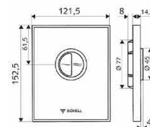
03 073 00 99 SCHELL cisterna MONTUS C 120 n para obra de fábrica DN 15 R 1/2".
